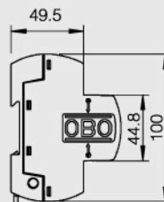
MCD 50-B尺寸图
