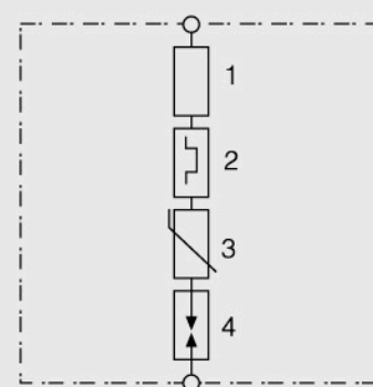
V20-VA结构图
