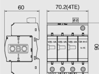
V20-VA尺寸图
